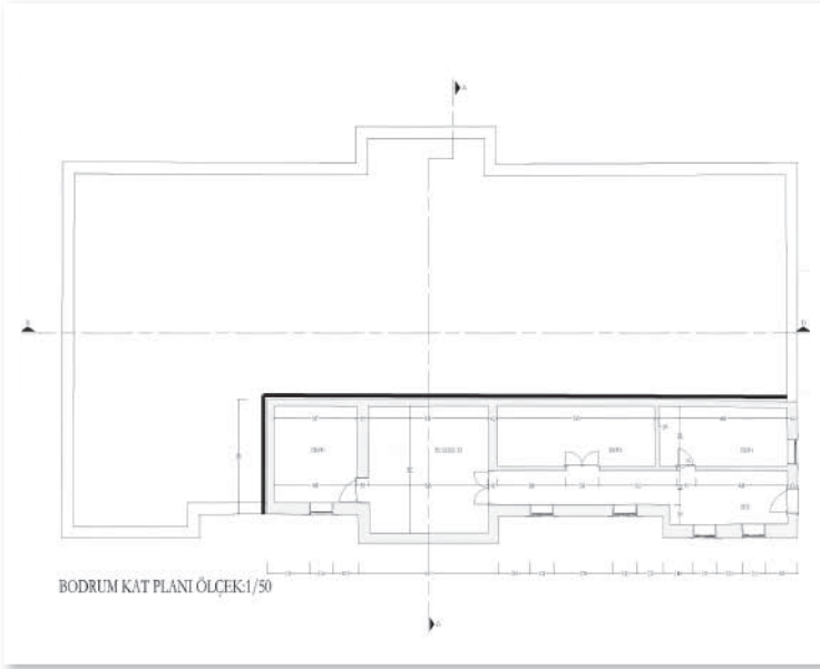
Çizim-1: Niksar Hükümet Konağı Bodrum Kat Planı (Niksar Belediyesi Arşivi)
