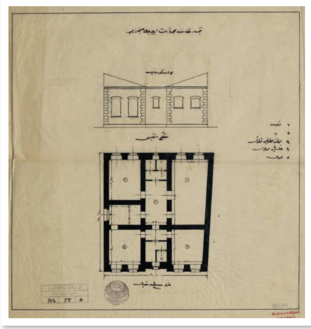
Çizim-3: Niksar Hapishanesi Proje ve Ön Cephe Görünüşü Yeniden Düzenlenmiş Hâli (Kaynak: BOA, DH.MB. HPS, nr. 112/55/6.).
